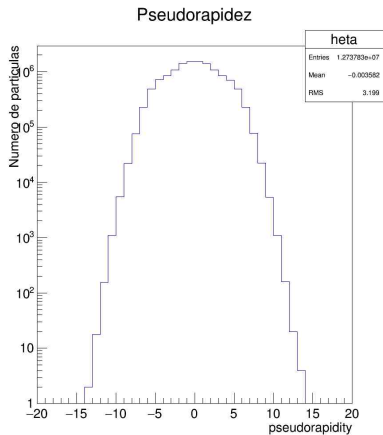
Figura: Pseudorapidez todas
