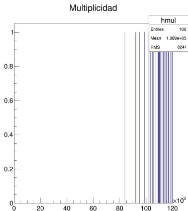
Figura: Multiplicidad \pi^-
