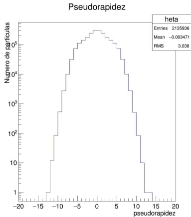
Figura: Pseudorapidez \pi^-
