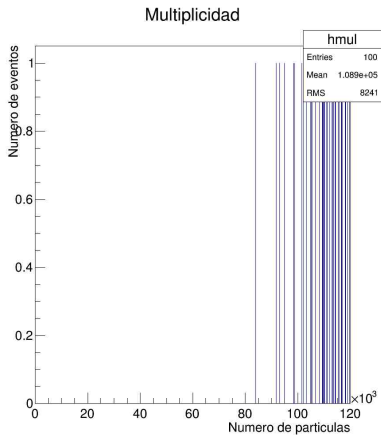
Figura: Multiplicidad todas
