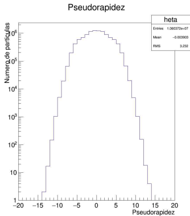
Figura: Pseudorapidez \eta
