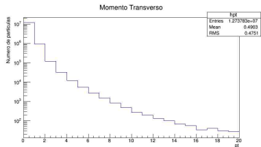
Figura: Momento todas
