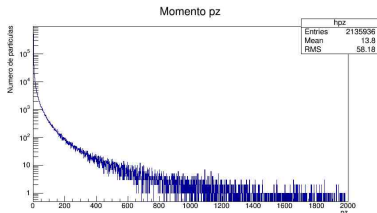
Figura: Momento pi^-
